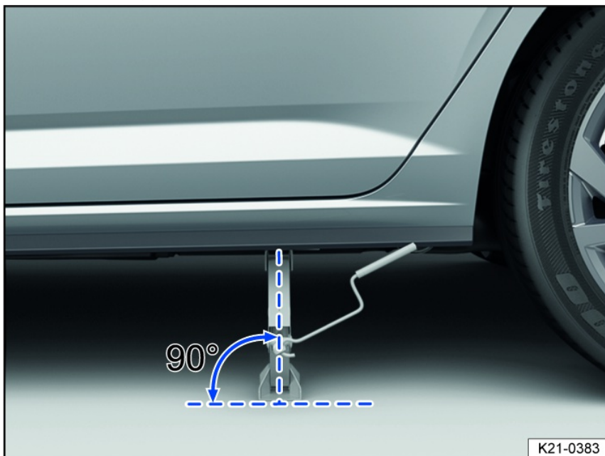
Fig. 180 Correct jack setup (variant 2).
